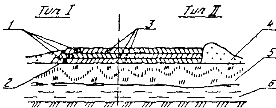
Рис. 1. Усиление ледового покрова методом послойного намораживания льда 1 - притрамбованный снег; 2 - жерди; 3 - намораживаемые слои; 4 - валик из снега; 5 - естественный ледяной покров; 6 - вода
