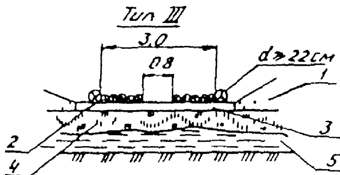
Рис. 2. Усиление ледовых переправ деревянным настилом 1 - снеговой покров; 2 - колесопроводы; 3 - поперечины; 4 - естественный ледяной покров; 5 - вода
